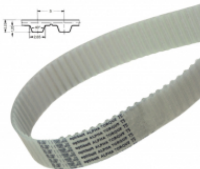
PAS ZĘBATEY T5
