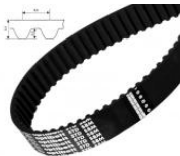
PAS ZĘBATY S8M
