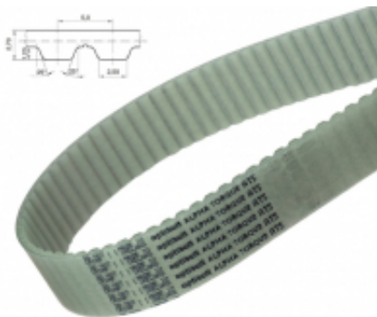
PAS ZĘBĄTY AT5
