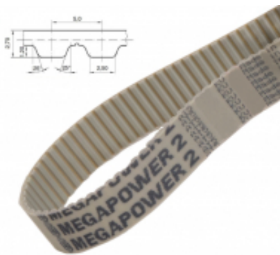
PAS ZĘBATY OTWARTY AT5 KV
