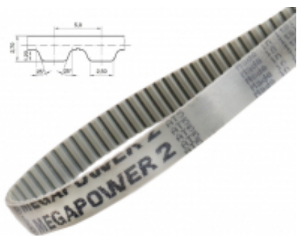
PAS ZĘBATY OTWARTY AT5
