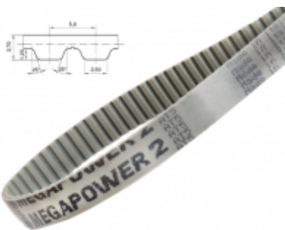
PAS ZĘBATY OTWARTY AT5
