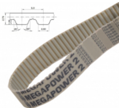
PAS ZĘBĄTY OTWARTY AT5 KV
