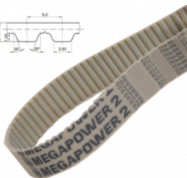
PAS ZĘBATY OTWARTY AT5 KV
