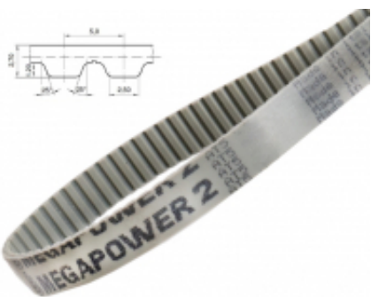
PAS ZĘBATY OTWARTY AT5
