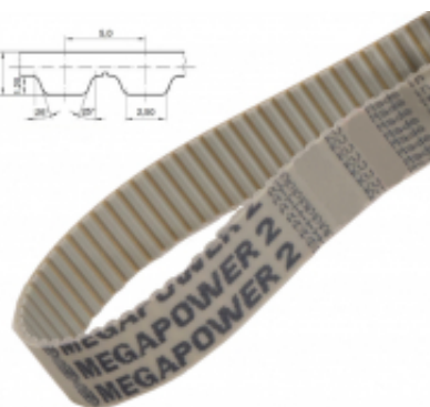
PAS ZĘBATY OTWARTY AT5 KV
