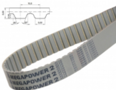
PAS ZĘBATY AT10 KV
